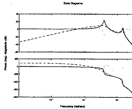
Fig. 5. Direct approach: P_0 (—), \hat{P} (---), T_{12} (-·-) and T_{22}H_0 (···)
